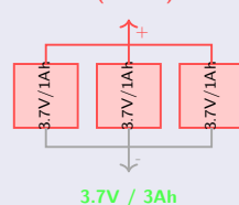
1S3P (Parallel)
